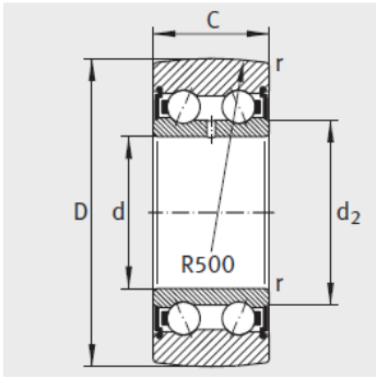
LR50...-2RS、LR52...-2RS、 LR53...-2RS
