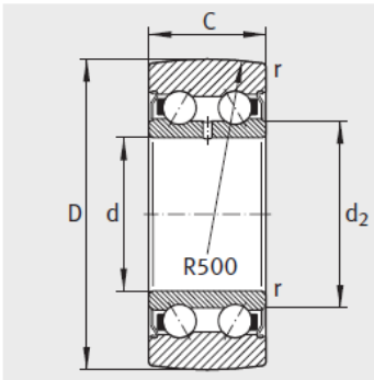
LR52...-2Z、LR53...-2Z、 LR52...-X-2Z 1)
