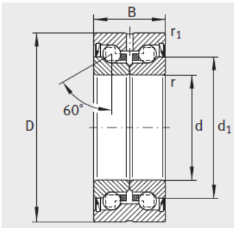
ZKLN..-2RS-PE
