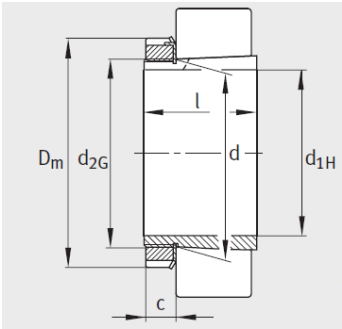
锥度为 1：12（H240、H241 系列，锥度为 1：30） 止动垫圈 MB、MBL
