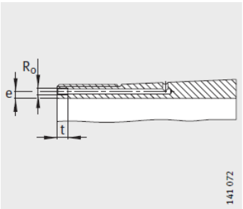
液压紧定套（后缀 HG） 安装尺寸
