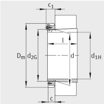
锥度为 1：12 (H240 系列，锥度为 1：30) 止动卡板 MS30
