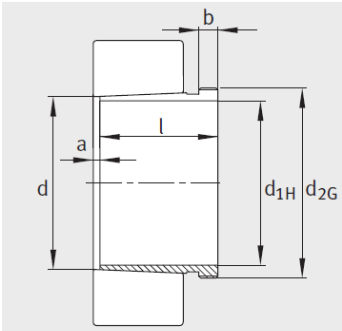
AH240、AH241 锥度为 1：30
