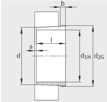
锥度为 1：12
