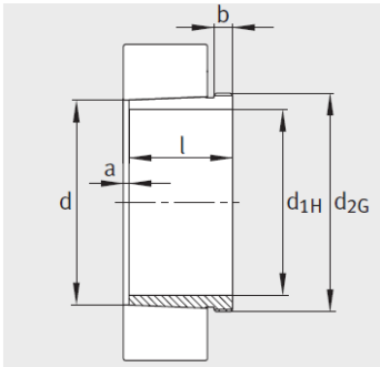
锥度为 1：12
