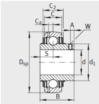
GYE12-KRR-B-VA
