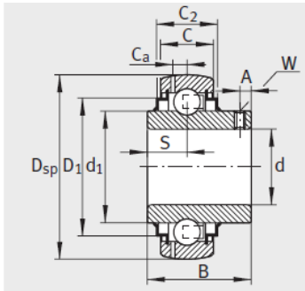
GYE12-KRR-B
