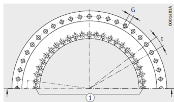
孔的分布 ① 两个保持螺栓
