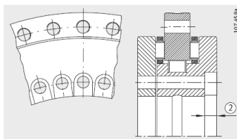
对于 YRT80-TV 和 YRT100 : ② 螺栓沉头孔开口方向 5)
