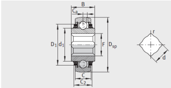
GVK...-KTT-B(AH...)-AS2/V、 VK...-KTT-B(AH...)
