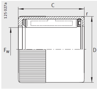
HF..-R、 HF..-KF-R 带滚花
